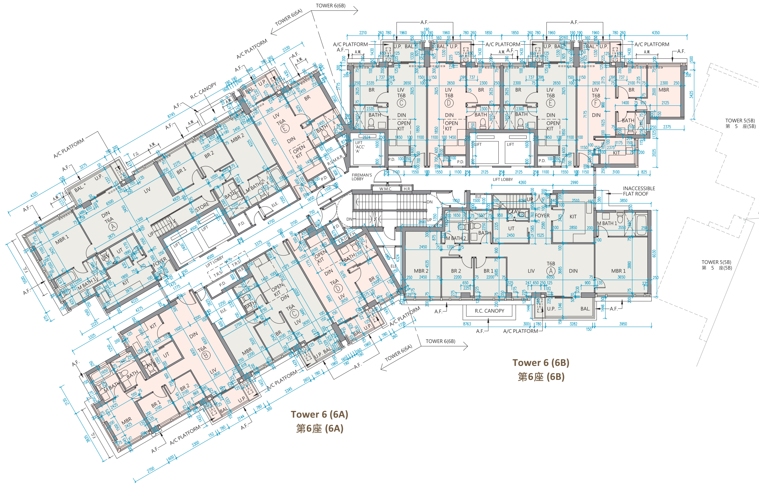
Tower 6 (6A) & Tower 6 (6B) | 28/F 第6座 (6A) 及第6座 (6B) | 28樓
